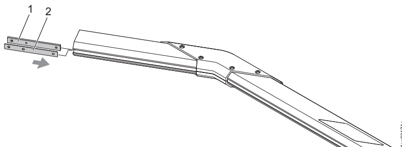
Rys. 52: Montaż wpustu przesuwneho i blachy dodatkowej
