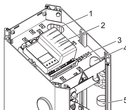
Rys. 43: Podłączenie przewodów sterowniczych
