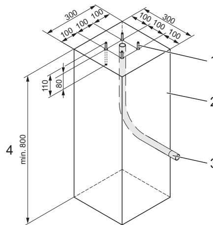
Rys. 17: Plan fundamentu słupka podporowego i słupka zapory świetlnej (wymiary w mm)
