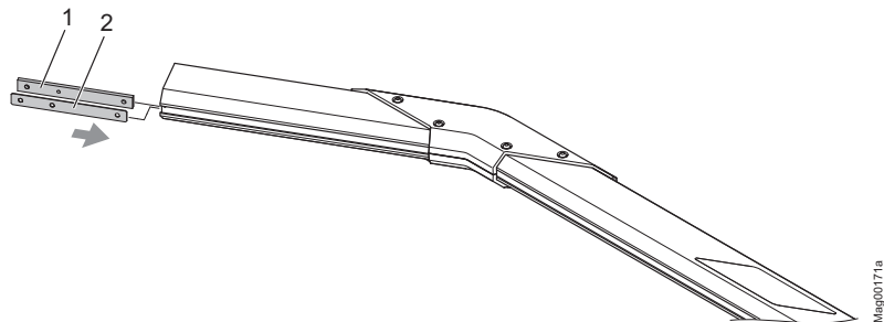
Rys. 26: Montaż wpustu przesuwnego i blachy dodatkowej
