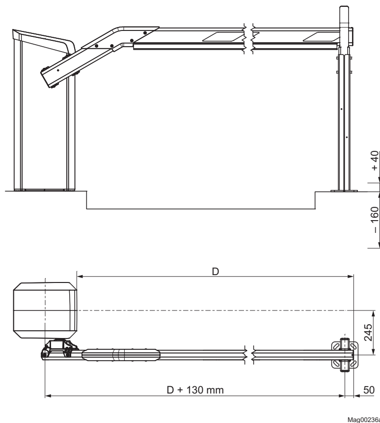
Rys. 16: Wymiary obudowy szlabanu – słupki (wymiary w mm)
