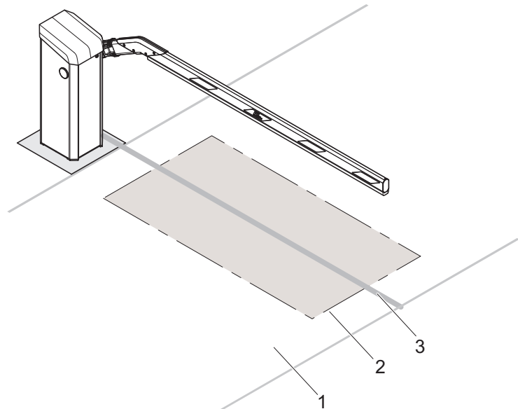
Rys. 18: Przykład umieszczenia pętli indukcyjnej dla ruchu samochodów osobowych, tu przedstawiony dla szlabanu typu "Access/Parking"
