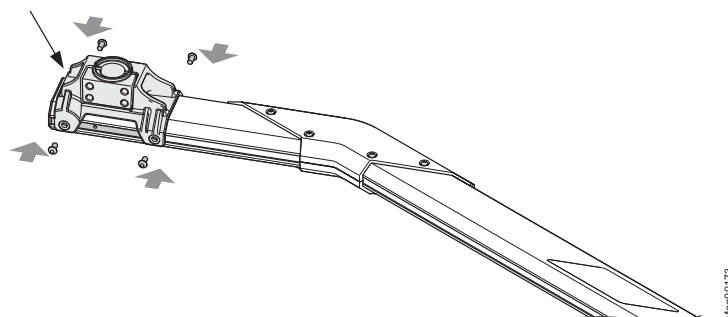
Rys. 54: Montaż kołnierza
