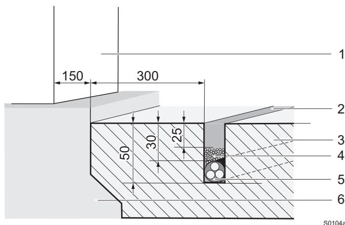
Rys. 20: Układanie pętli indukcyjnej w bitumie, asfalcie lub betonie (wymiar w mm)
