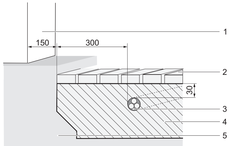
Rys. 21: Układanie pętli indukcyjnej pod nawierzchnią z kostki brukowej (wymiary w mm)
