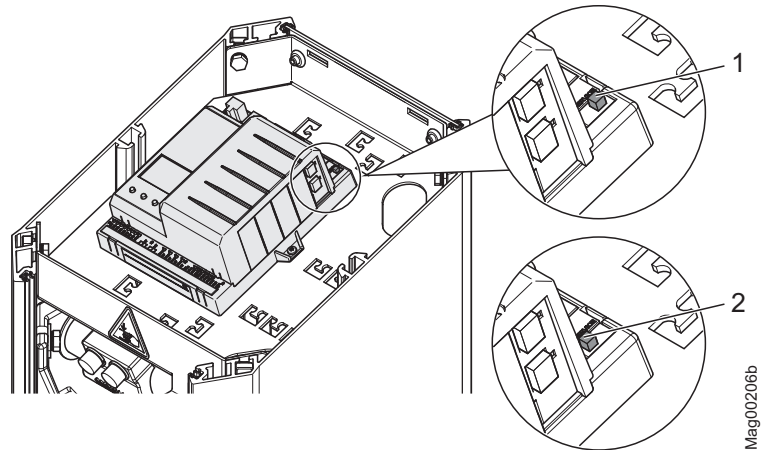
Rys. 47: Wyłącznik serwisowy
