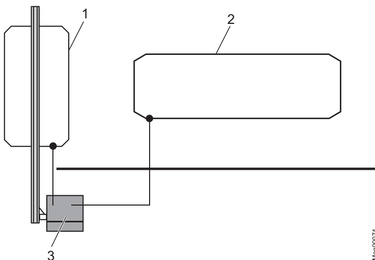
Rys. 9: Pętla dla samochodów osobowych – przejazd z długą pętlą otwierającą
