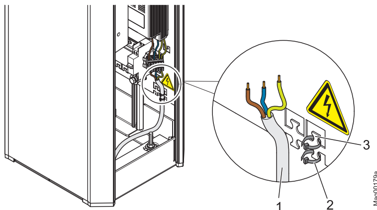
Rys. 41: Prowadzenie sieciowego przewodu zasilającego
