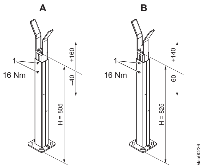
Rys. 38: Nastawianie wysokości słupka podporowego (wymiary w mm)
