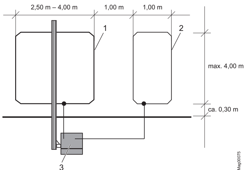
Rys. 10: Pętla dla samochodów ciężarowych
