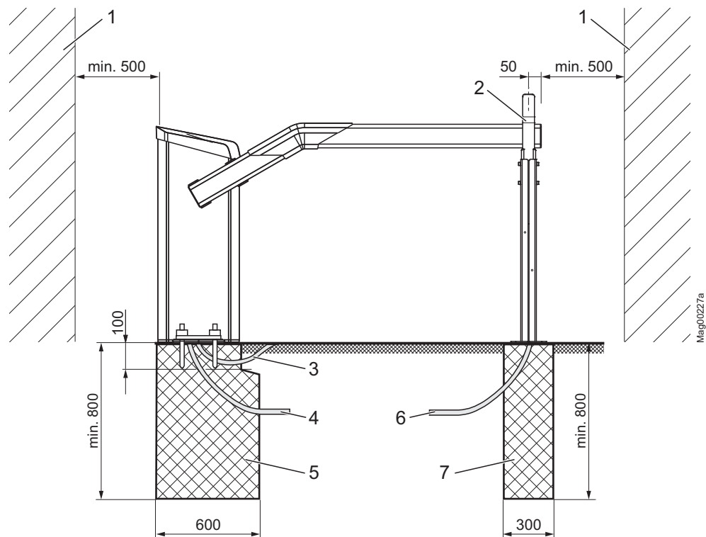
Rys. 13: Montaż szlabanu, tu przedstawiony dla szlabanu typu "Access/Parking" (wymiar w mm)
