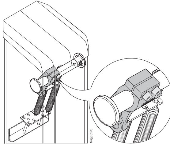
Rys. 34: Poluzowanie śrub z łbem walcowym o gnieździe sześciokątym przy dźwigni zaciskowej
